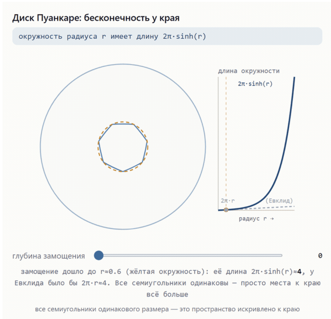
Рисунок 16.2. Диск Пуанкаре и рост длины гиперболической окружности.
