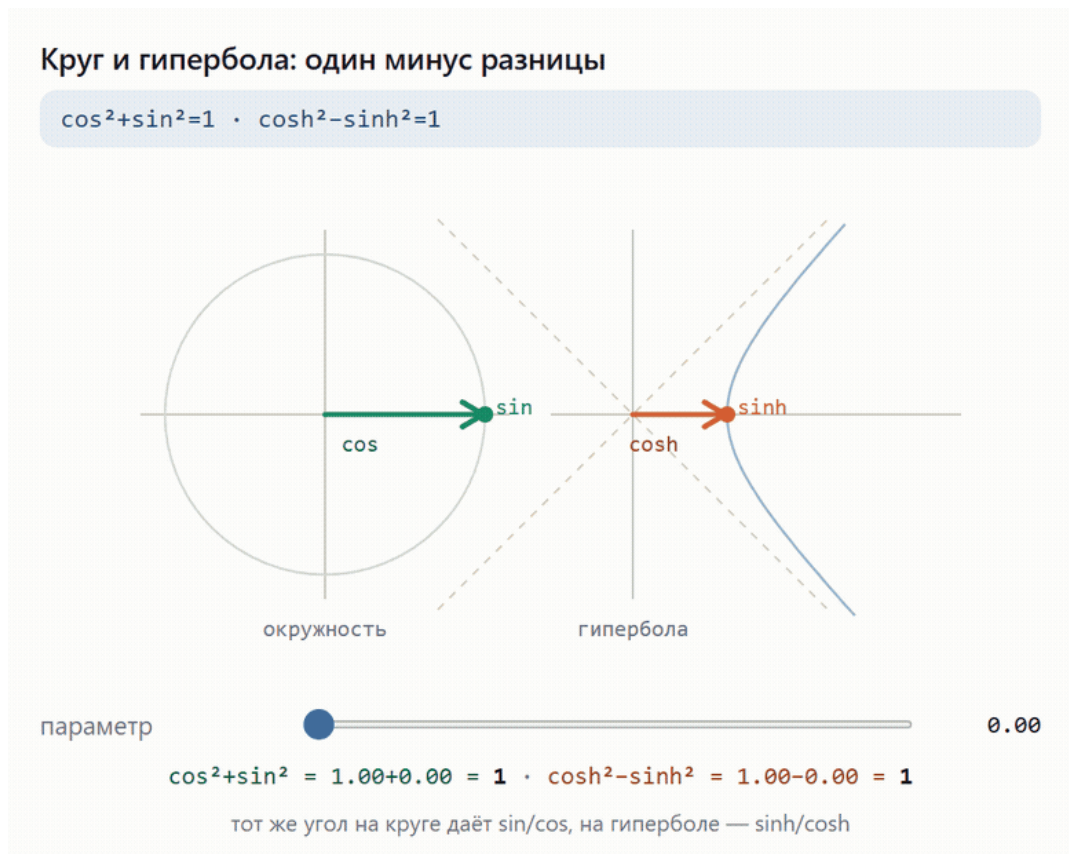
Рисунок 16.3. Компактная и некомпактная единичные квадрики: окружность и гипербола.
